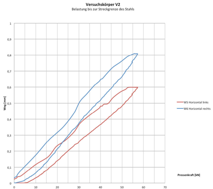
Bild 9 Verformungen Versuchskörper V2, horizontal über den Absorbern gemessen, Belastung bis zum Erreichen der Streckgrenze des Stahls
