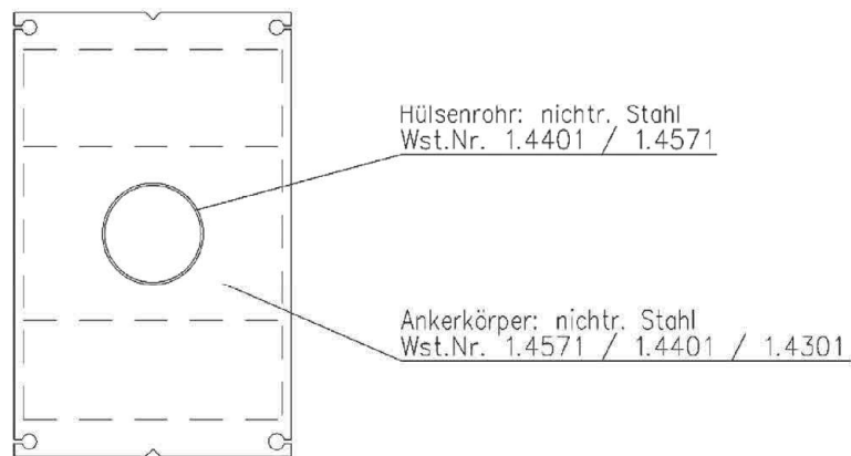
Teil Hülse DND
