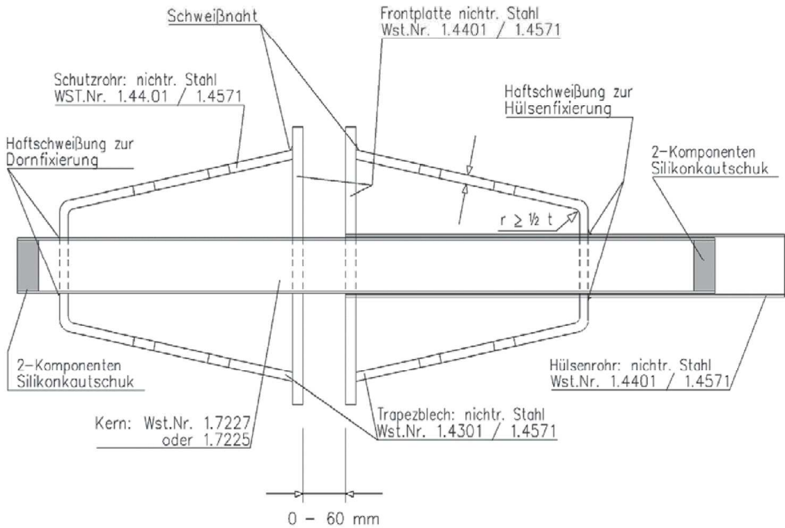
Teil Hülse DND
