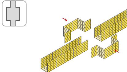
Fundament Erweiterungen
